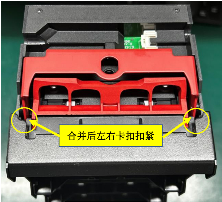
图二，将 PA4485-6 合上，并用 MC2503 手柄扣紧。
