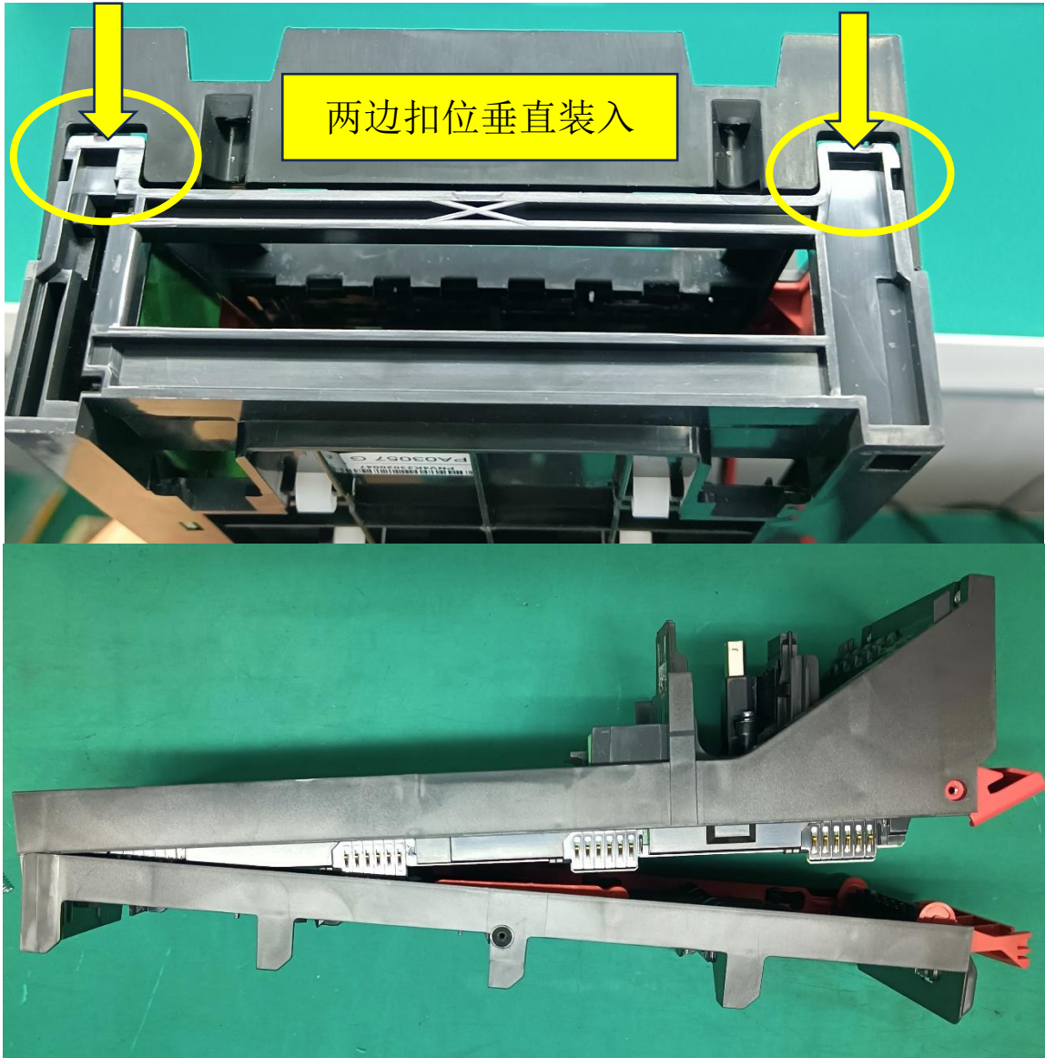
图一，将 PA3055 组件两边骨对准 PA4485-1 组件两边槽位装入
